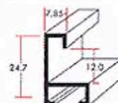
Алюминиевый багет, 1м.п. артикул № 10
