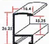
Алюминиевый багет, 1м.п. артикул № 901
