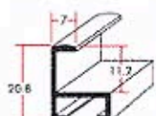
Алюминиевый багет, 1м.п. артикул № 11
