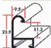
Алюминиевый багет, 1м.п. артикул № 88
