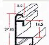
Алюминиевый багет, 1м.п. артикул № 19
