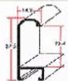
Алюминиевый багет, 1м.п. артикул № 64
